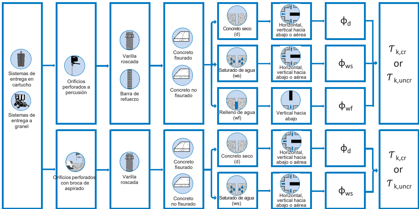
FIGURA 2 - Detalle de instalación típica para varilla roscada o barra de construcción
