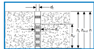
FIGURA 3 - Detalle de instalación típica para insertos internamente roscados
